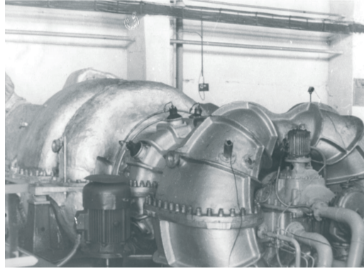
Первая турбина пущенная в работу ТКЦ №6 Палласовского ЛПУМГ, 1974 год
