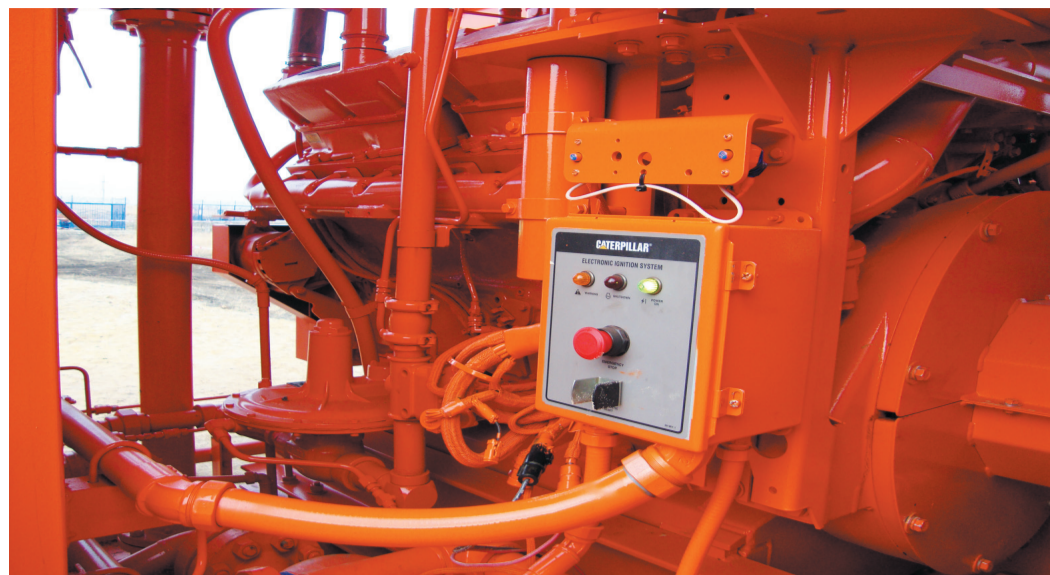
Двигатель МКУ
